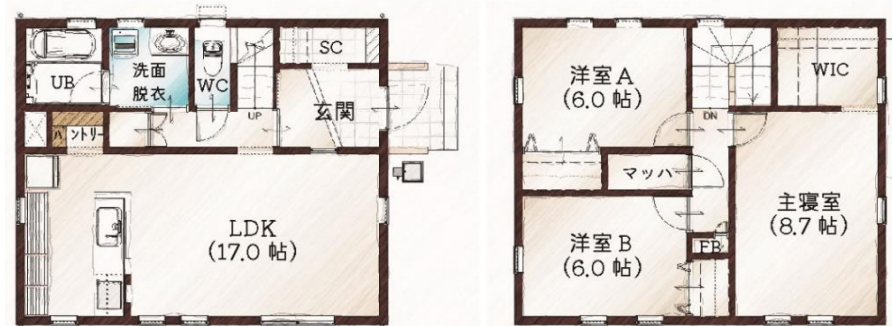
1階平面図
